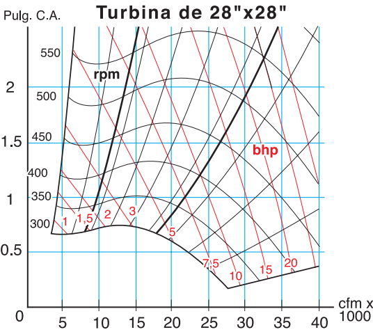
Curvas del ventilador, SNM. En estas gráficas no esta considerada la perdida por filtro y transmisión.
