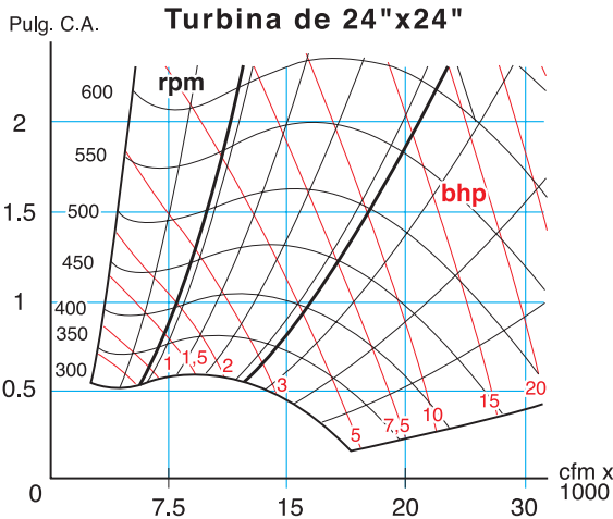
Curvas del ventilador, SNM. En estas gráficas no esta considerada la perdida por filtro y transmisión.
