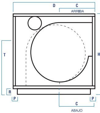
MODELOS MH DESCARGA HORIZONTAL
