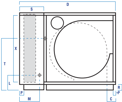
MODELOS MH DESCARGA HORIZONTAL
